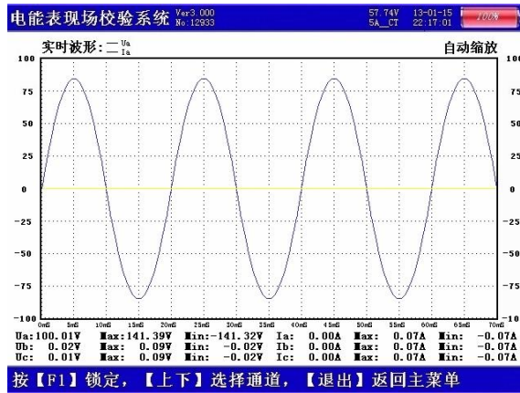
图十三、波形显示屏
