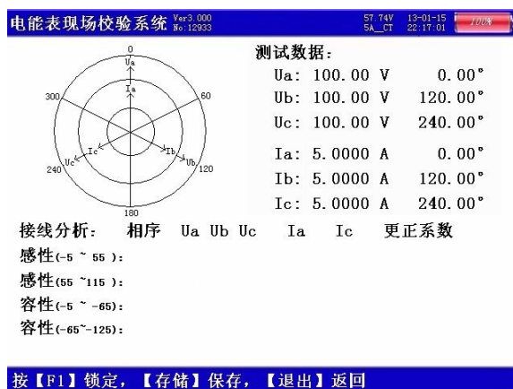
图九、矢量分析屏—三相四线
