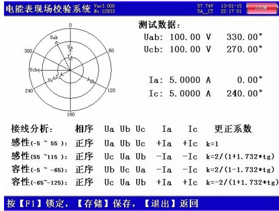
图十、矢量分析屏一三相三线
