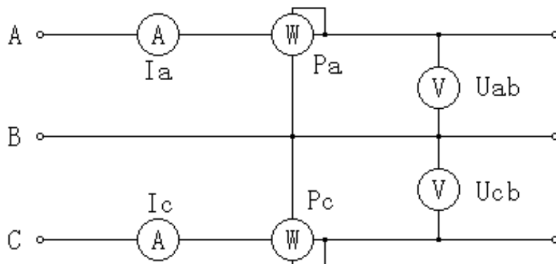
图十七、三相三线计量原理图
