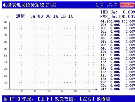
图十四、频谱分析屏
